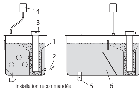
Installation recommandée
