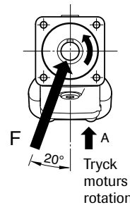
Optimal angreppsvinkel för radiallaster
